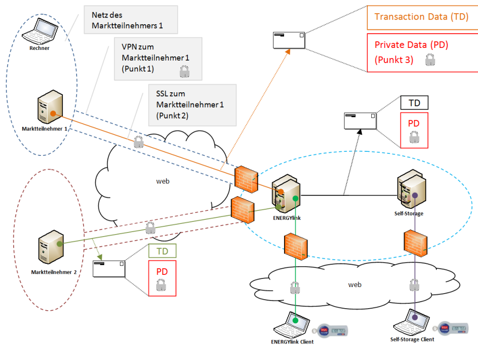
Abbildung 665 Sicherheitsebenen
