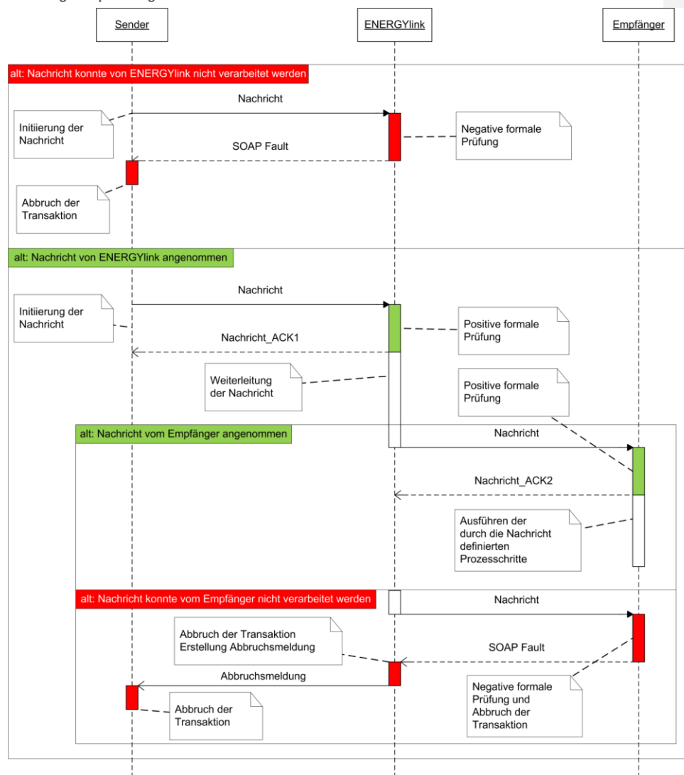
Abbildung 4 Sequenzdiagramm
