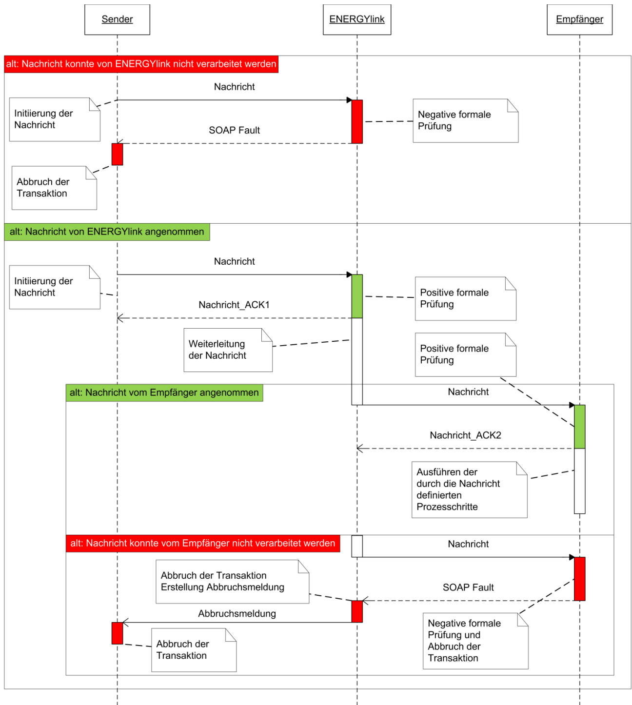
Abbildung 4 Sequenzdiagramm
