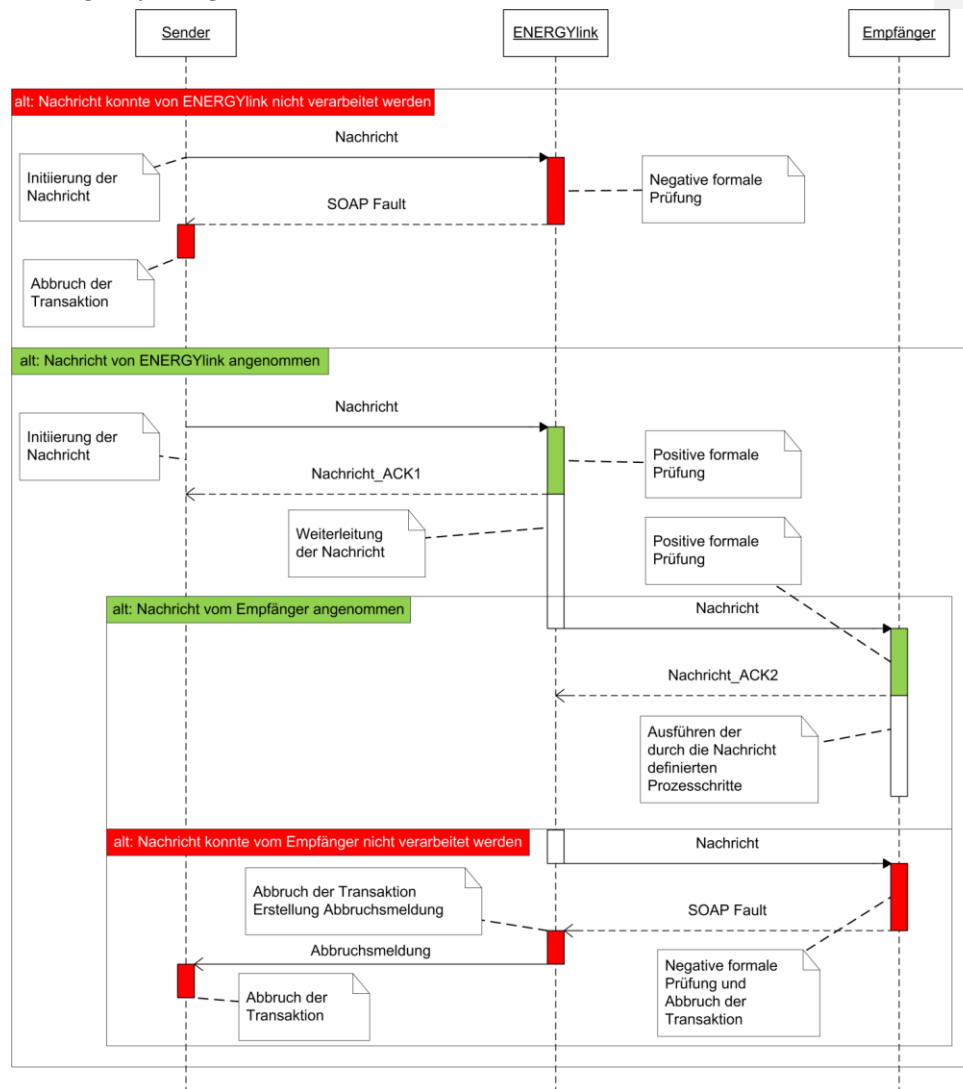
Abbildung 4 Sequenzdiagramm
