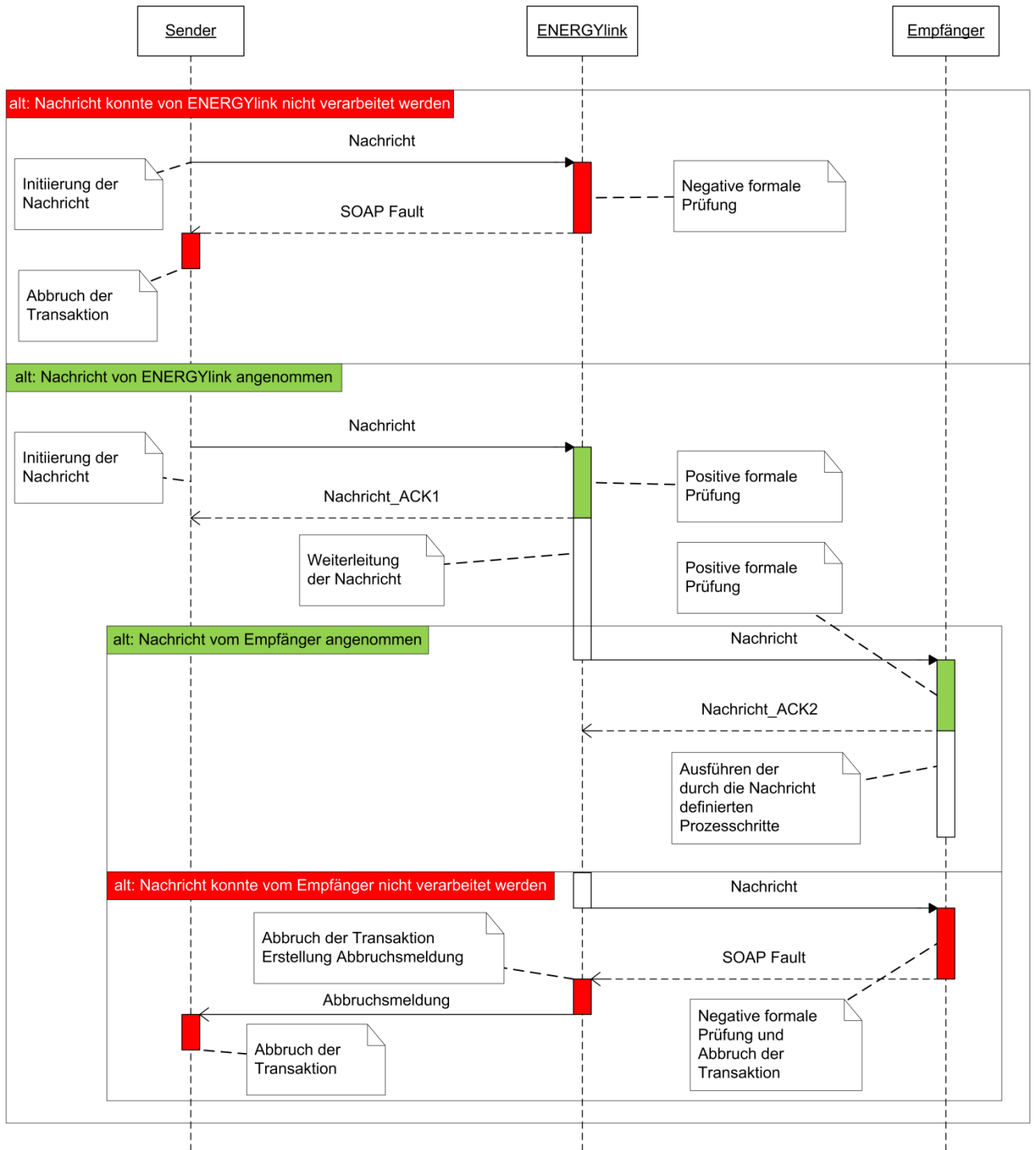
Abbildung 4 Sequenzdiagramm
