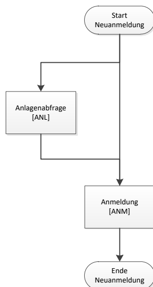
Abbildung 23: Überblick Anmeldeverfahren
