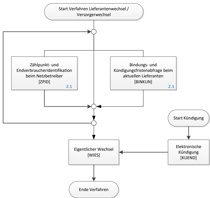
Abbildung 1: Überblick Lieferantenwechsel
